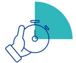
Tijdsregistratie app
