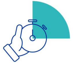
Tijdsregistratie app
